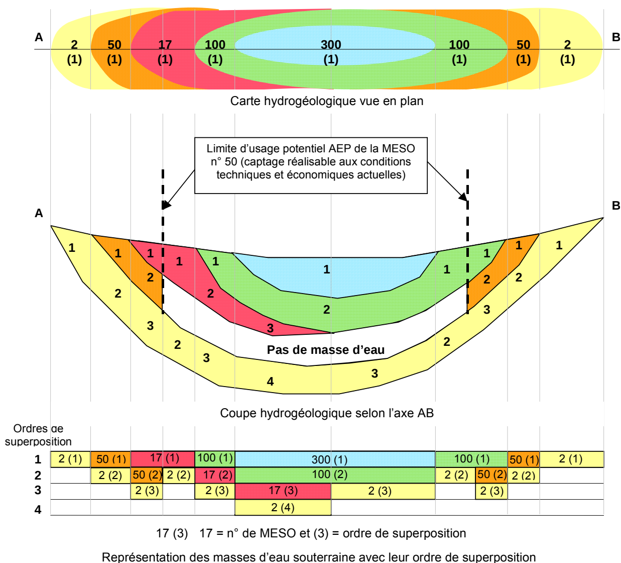
Figure 2 : Schéma de principe de la superposition des masses d'eau souterraine
