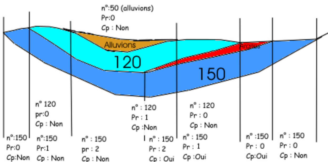
Figure 7 : Coupe hydrogéologique schématique avec 3 masses d'eau souterraines superposées (n° 50, 120 et 150)
