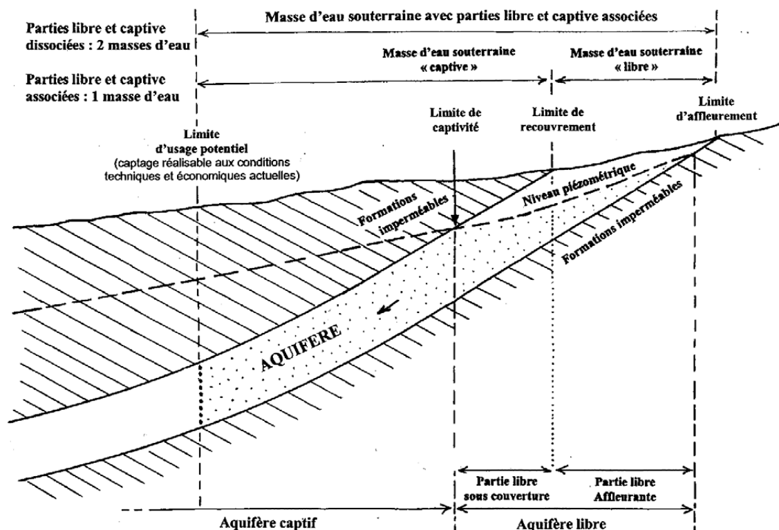
Figure 1- Limites des parties libre et captive d'une masse d'eau souterraine de type dominante sédimentaire non alluviale (vue en coupe)
